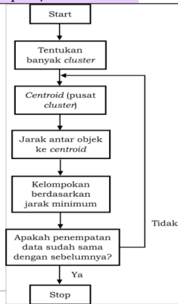
Gambar 1. Tahapan Analisis Kluster Metode K-Means
