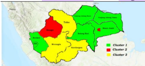
Gambar 2. Persebaran Klaster Berdasarkan Peta Provinsi Jambi
