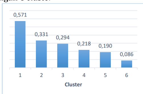
Gambar 2. Rata-rata per klaster
