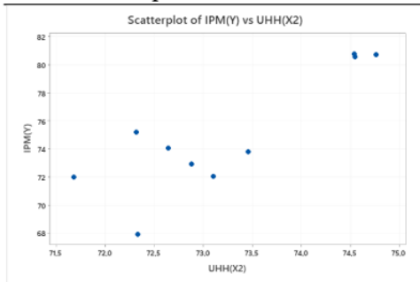
Gambar 2. Scatterplot Variabel Y Terhadap X 2
