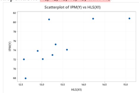
Gambar 1. Scatterplot Variabel Y Terhadap X_1
