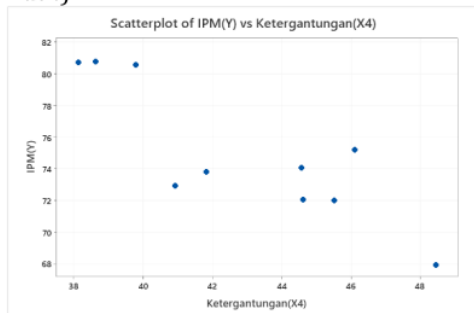
Gambar 4. Scatterplot Variabel Y Terhadap X 4
