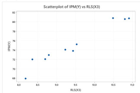
Gambar 3. Scatterplot Variabel Y Terhadap X 3
