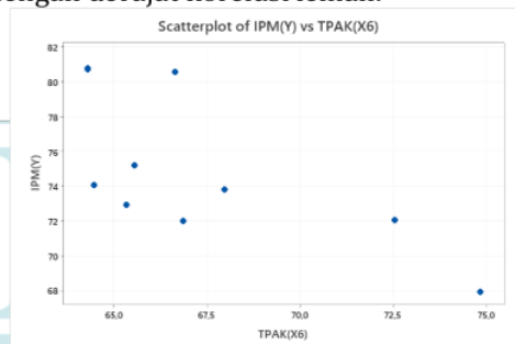
Gambar 6. Scatterplot Variabel Y Terhadap X 6
