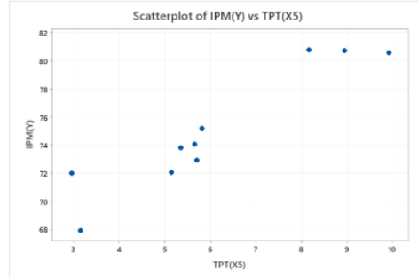
Gambar 5. Scatterplot Variabel Y Terhadap X 5
