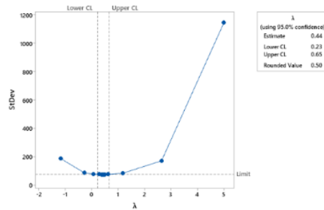
Gambar 4. Box-Cox Curah Hujan
