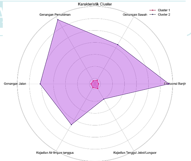
Gambar 6. Karakteristik Cluster
