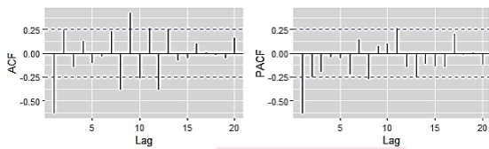
Gambar 3. Plot ACF dan PACF
