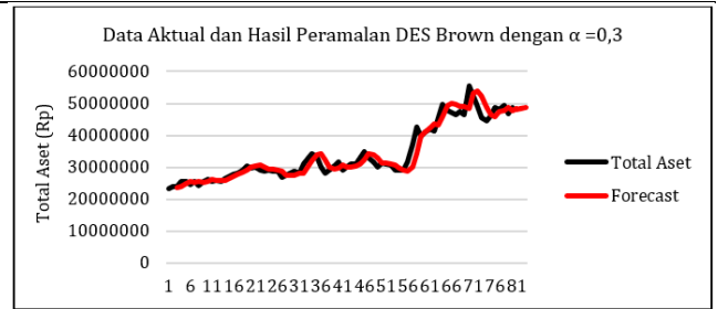
Gambar 3. Grafik Perbandingan Data Aktual dengan Hasil Peramalan.
