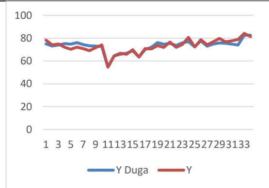
Gambar 3. Plot Y dan Y Duga Spline Truncated
